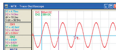
Anzeige mit Nachleuchtdauer beim MTX 162
