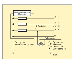
Prinzip der Schleifenwiderstandsmessung / Neutralleiter liegt auf Erde
